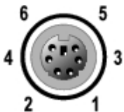
Figura B-4. Números de patas del conector para teclado
