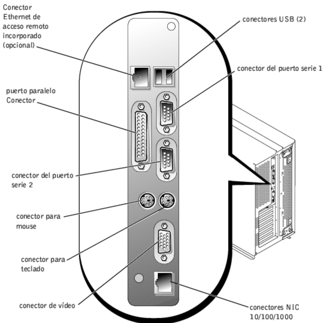
Figura B-1. Puertos y conectores de E/S del panel posterior
