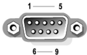
Figura B-2. Números de patas del conector de puerto serie
