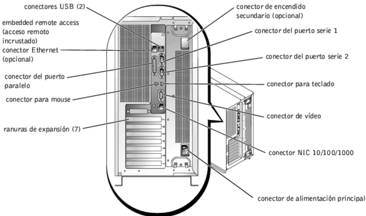
Figura 1-6. Características del panel posterior
