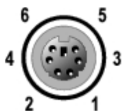
Figura B-5. Números de patas en el conector para mouse
